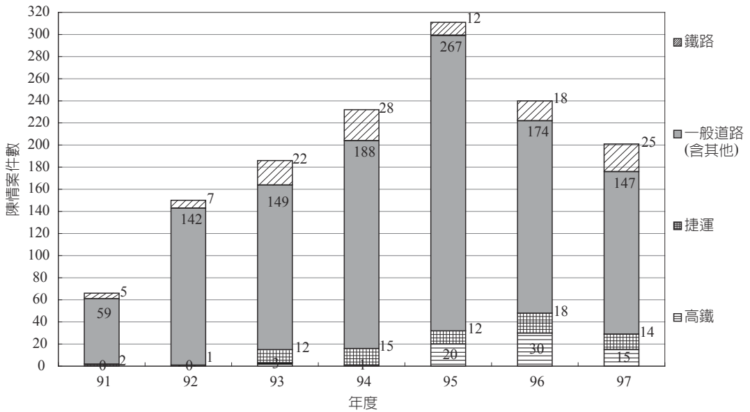
圖 3.2-2 我國91年至97年交通噪音陳情案件統計圖
