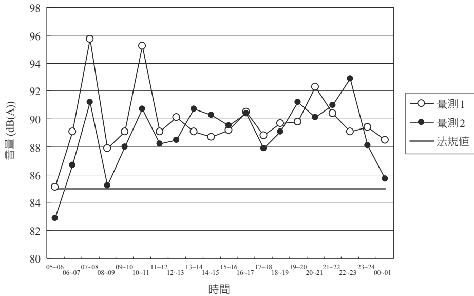
圖 3.1-11 台灣一般鐵路 L_{max, mean, 1h} 量測結果示意圖
