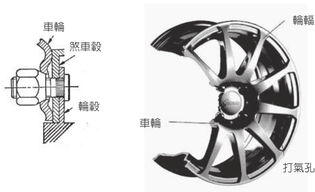
圖 3.3-2 輪轂 (wheel hub) 與輪輻 (spoke) 示意圖
