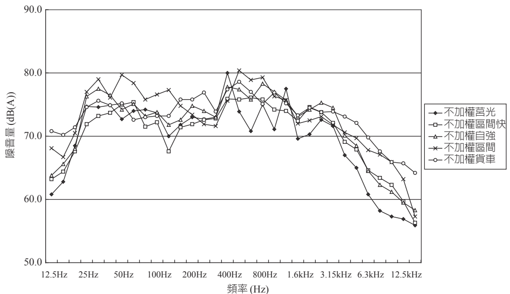
圖 3.1-2 我國鐵路噪音頻譜圖
