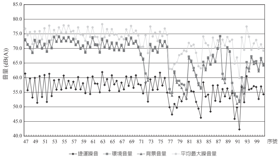
圖 3.1-8 台北捷運木柵線各站監測結果
