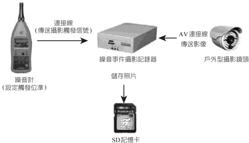
圖 3.2-3 噪音事件攝影記錄系統架構圖
