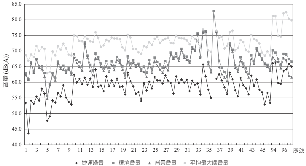
圖 3.1-7 台北捷運淡水線各站監測結果
