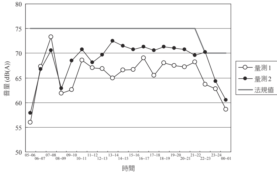
圖 3.1-10 台灣一般鐵路 L_{eq,1h} 量測結果示意圖
