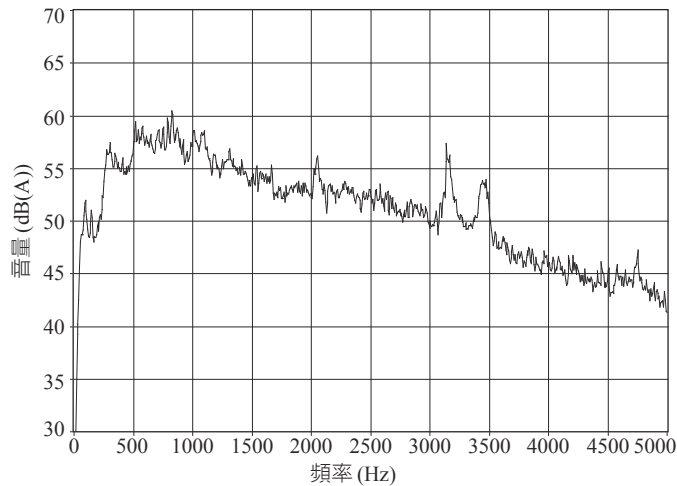
圖 3.1-5 我國高速鐵路噪音頻譜
