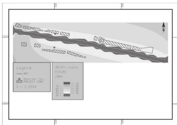
圖 3.2-7 SoundPlan 音場 L_{max, mean, 1h} 模擬平面示意圖
