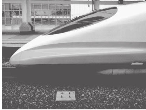
圖 3.3-3 隔音裙
