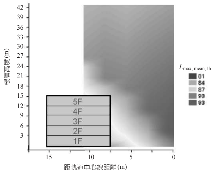
圖 3.2-5 SoundPlan 音場模擬剖面示意圖
