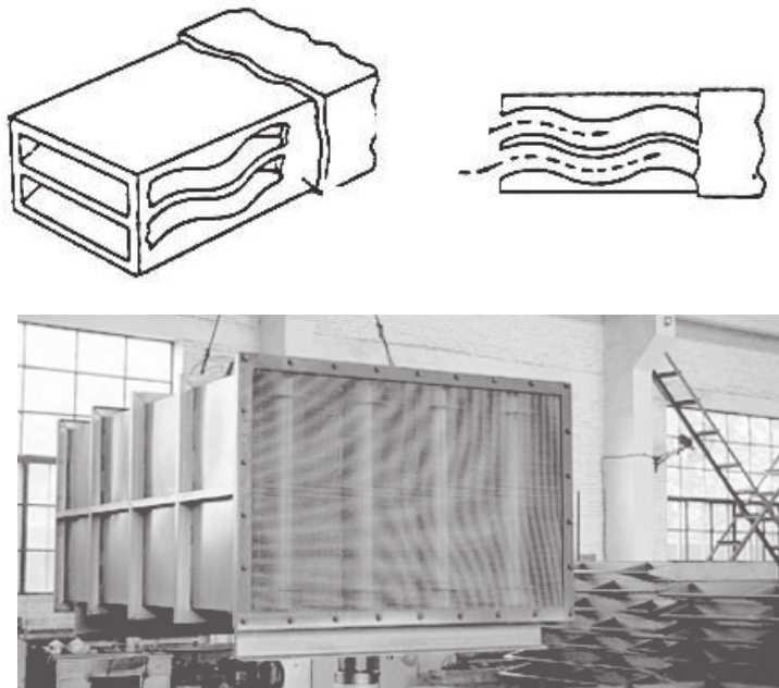
圖 10.1-4 折板式消音器
