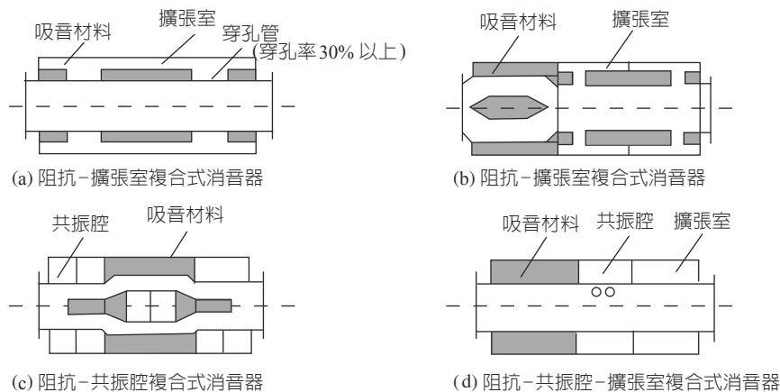
圖 10.3-1 常見的阻抗複合型消音器
