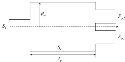
圖 10.4-4 雙出口擴張室消音器
