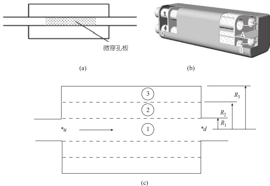
圖 10.3-2 (a) 單層微穿孔板，(b) 多微穿孔板並行結構 3D 模型，(c) 多層微穿孔板結構
