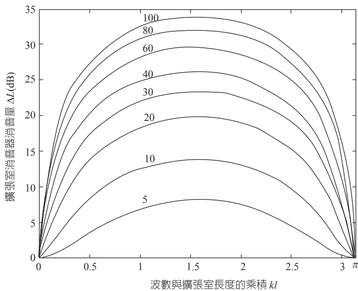
圖 10.2-3 單節擴張室消音器以擴張比為參數的消音量
