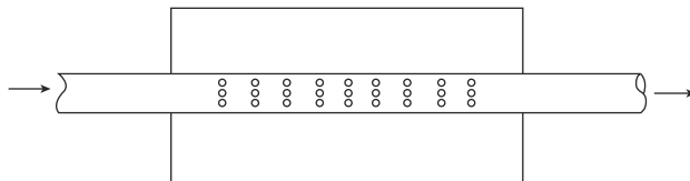
圖 10.2-6 單腔共振腔消音器
