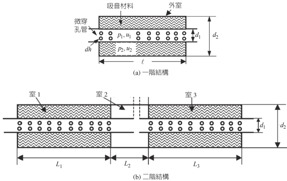
圖 10.3-4 阻性 - 微穿孔複合消音器
