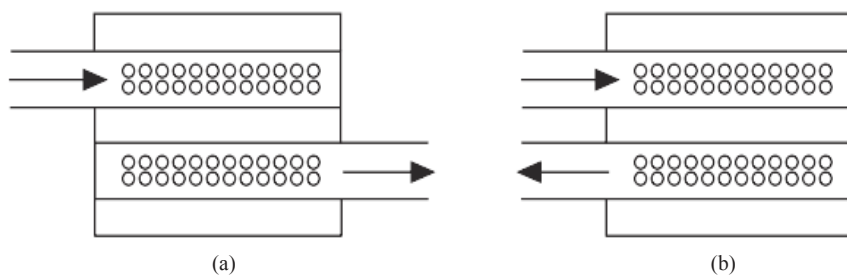
圖 10.3-3 (a) 錯流消音器，(b) 錯 - 回流消音器
