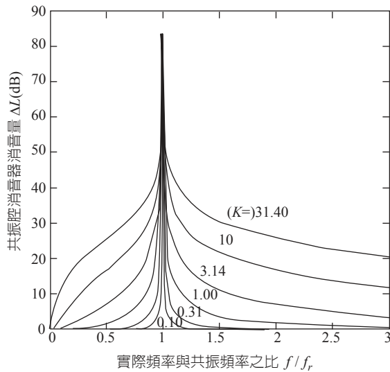
圖 10.2-7 共振腔消音器以 K 值為參數的消音性能曲線
