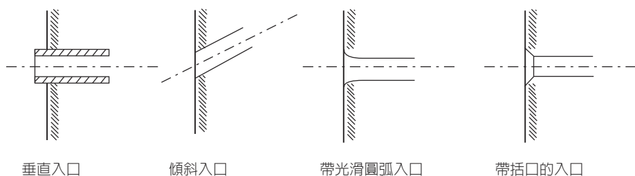
圖 10.4-1 幾種常見入口形式
