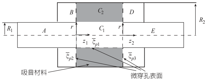
圖 10.3-5 改進的阻性 - 微穿孔複合消音器
