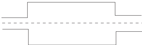
圖 10.2-2 單節擴張室消音器結構及消音特性示意圖
