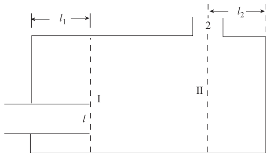
圖 10.2-4 直進 - 旁出的長擴張室消音器
