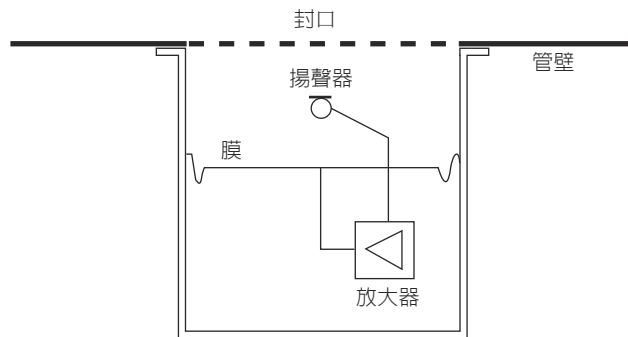
圖 10.3-8 有源（主動控制）消音器
