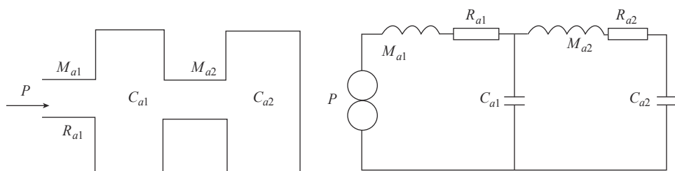
圖 10.2-1 抗性消音器的音類比
