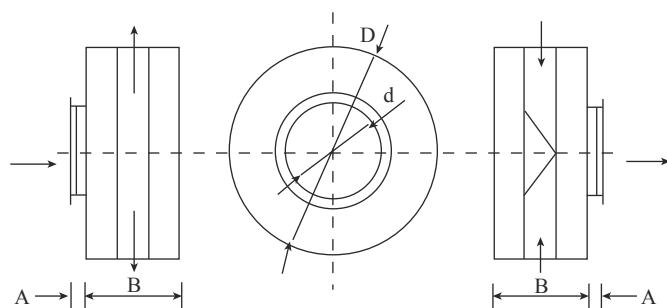
P型盤式消音器結構外形圖
