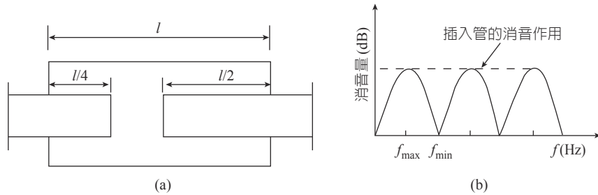
圖 10.2-5 (a) 帶內插管的擴張室消音器，(b) 內插管的作用
