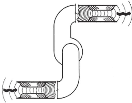
圖 10.3-6 小孔消音器
