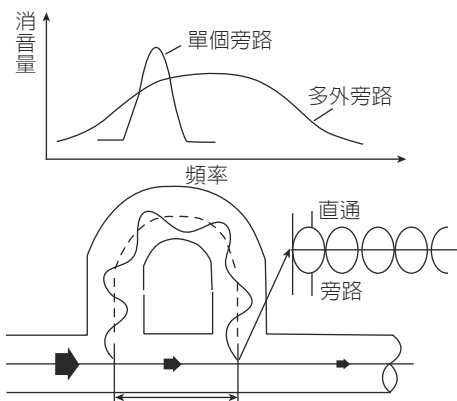
圖 10.3-10 干涉型消音器原理示意圖
