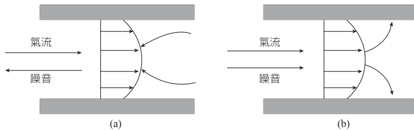
圖 10.4-3 (a) 氣流與音傳播反向時的折射，(b) 氣流與音傳播同向時的折射
