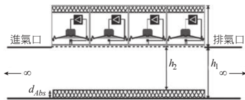
圖 10.3-9 有源 - 阻性混合消音結構
