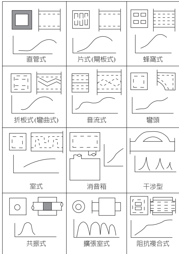
圖 10.1-1 幾種消音器及其頻譜特性示意圖
